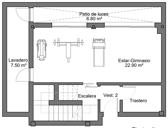
Planta sótano
